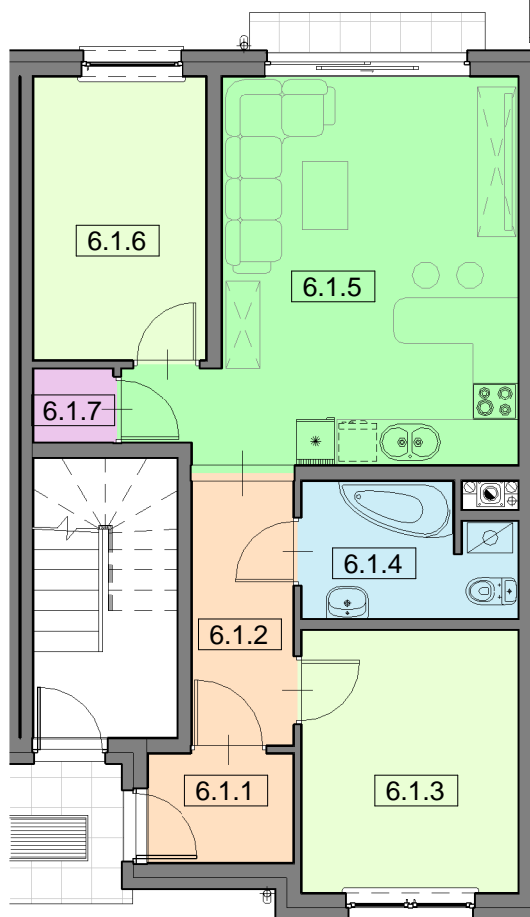
1 LOKAL 6.1 - PRZYZIEMIE 1 : 100
