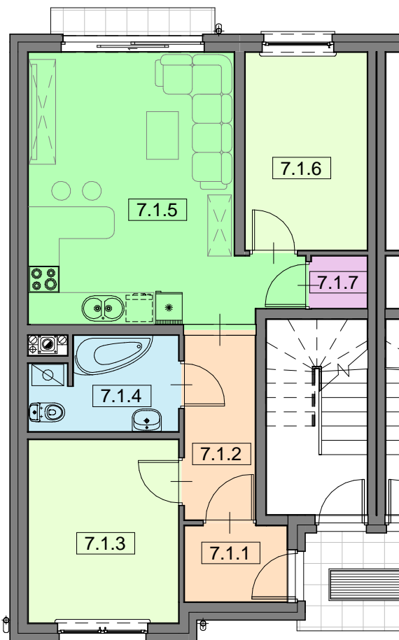
1 LOKAL 7.1 - PRZYZIEMIE 1 : 100
